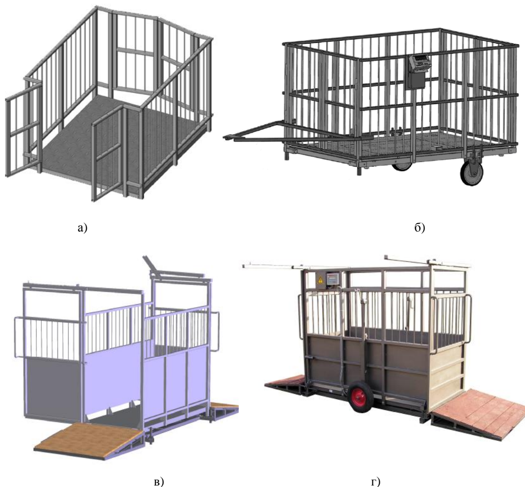
Рисунок 3 – Внешний вид весов с платформой с ограждением для взвешивания скота
