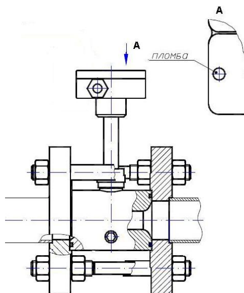
Рисунок 1 – Схема пломбирования датчика расхода газа ДРГ.М-160/80
