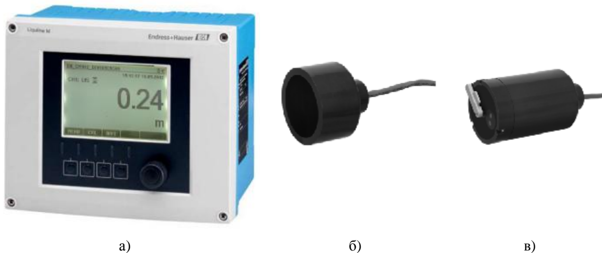
Р и с у н о к 1 – Уровнемеры ультразвуковые CM44x/CUS71D: а) контроллер CM44x, б) стандартный датчик уровня CUS71D, в) датчик со щёткой-очистителем CUS71D.
