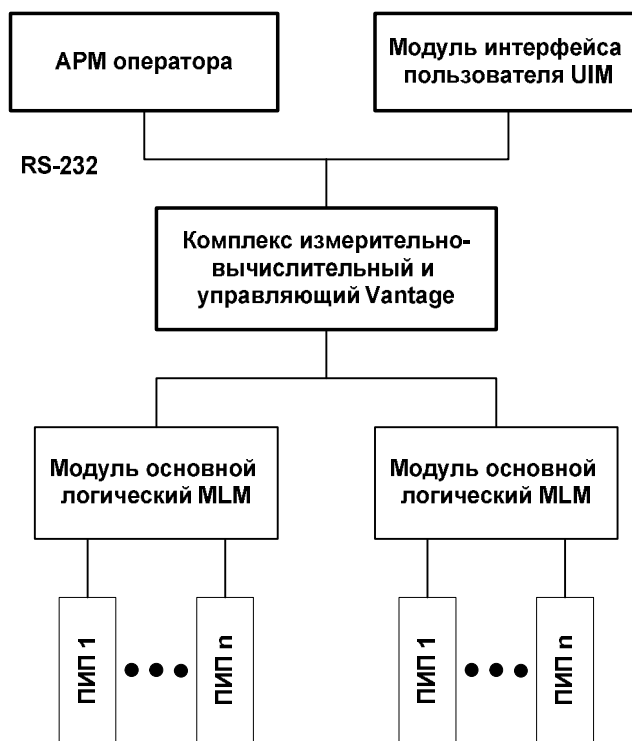
ПИП – первичный измерительный преобразователь Рисунок 1 – Структурная схема ИС
