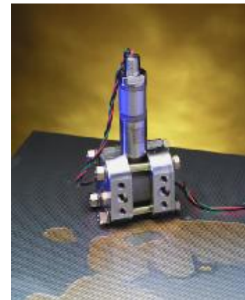
Рисунок 12 – Общий вид преобразователей модели 574
