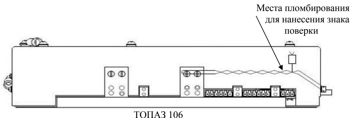
Рисунок 6 - Схемы пломбирования защитной крышки тумблера «Настройка/работа» отсчетного устройства БИУ
