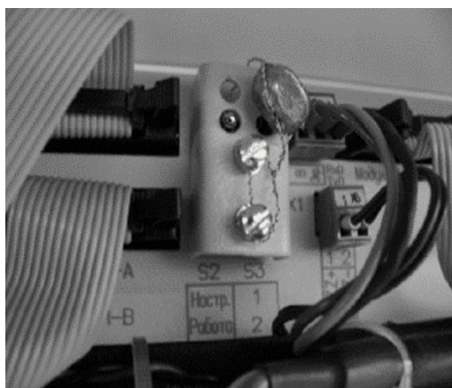
Рисунок 4 - Схемы пломбирования измерителей объема поршневых с датчиками импульсов
