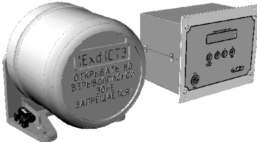
Рис.1 Фотография общего вида газоанализаторов ГТМК-18
