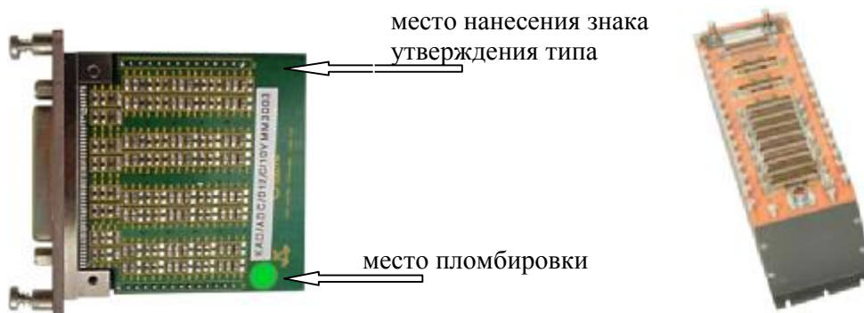
Рисунок 1 - Внешний вид модуля KAD/ADC/012 и модуля KAD/ADC/012 установленного в блок базовый KAM/CHS/13U
