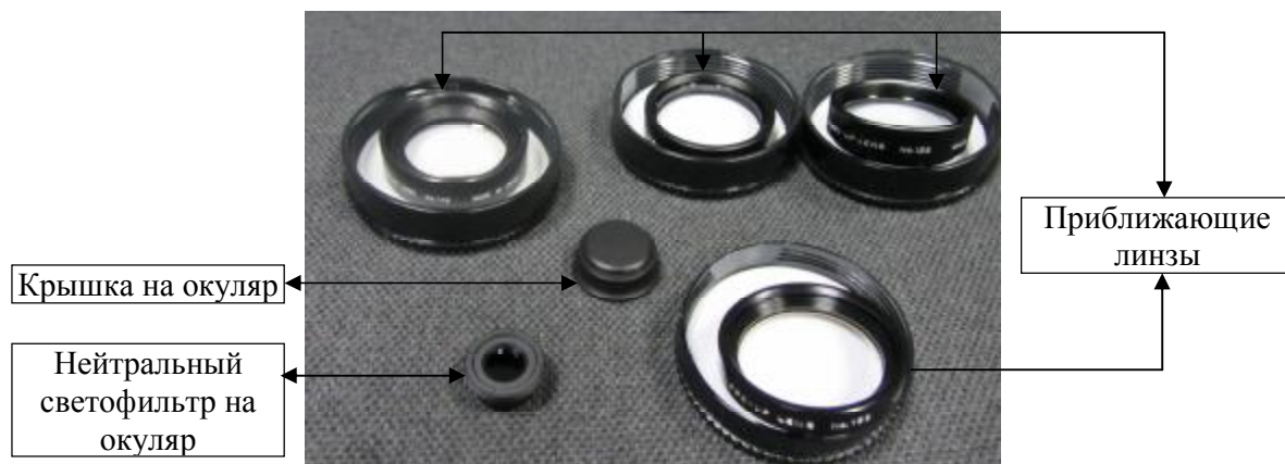
Рисунок 3 – Комплектующие яркомера LS-110
