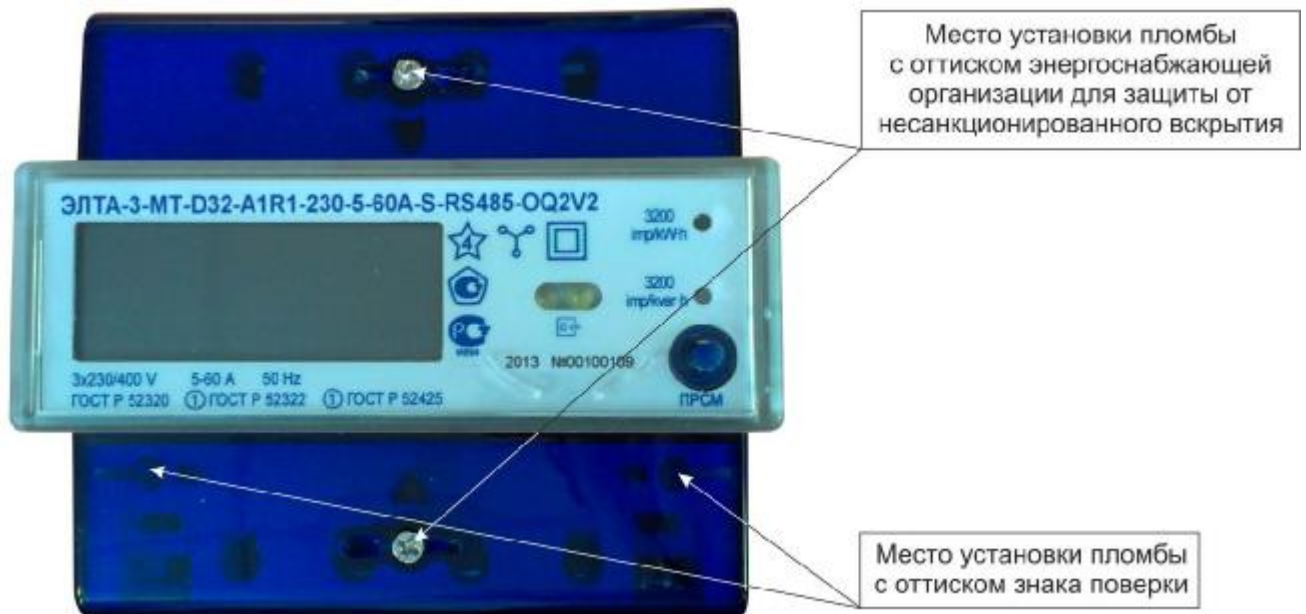
Рисунок 4 – Общий вид счетчика в корпусе модификации D32
