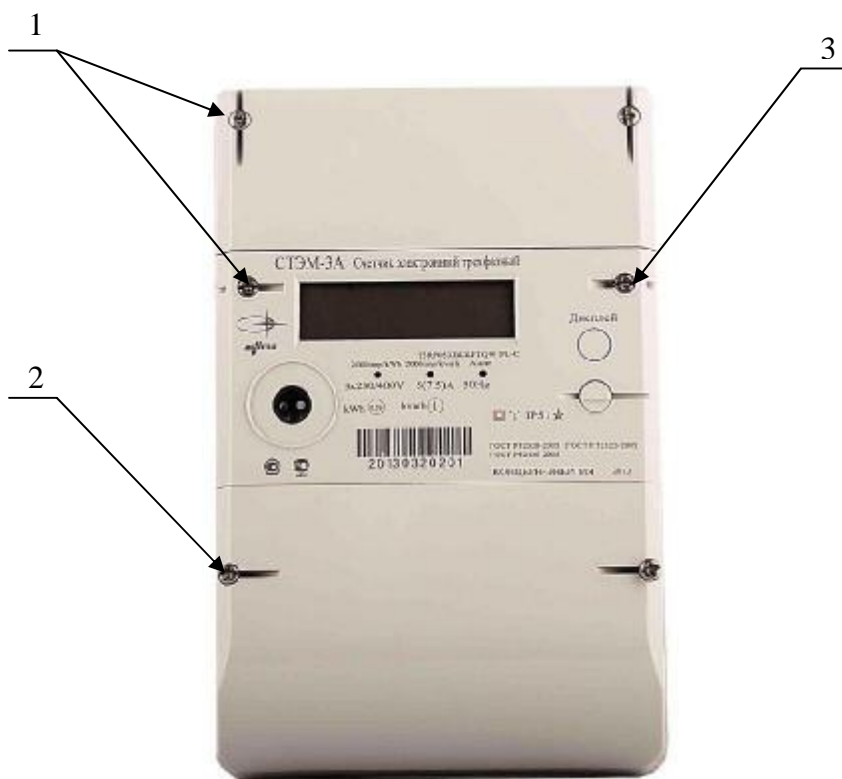
Рисунок 2 – Фотография общего вида счетчиков электрической энергии однофазных многотарифных СТЭМ-3А трансформаторного включения, где 1 – пломба ОТК завода-изготовителя; 2 – пломба энергоснабжающей организации; 3 – пломба поверяющей организации.
