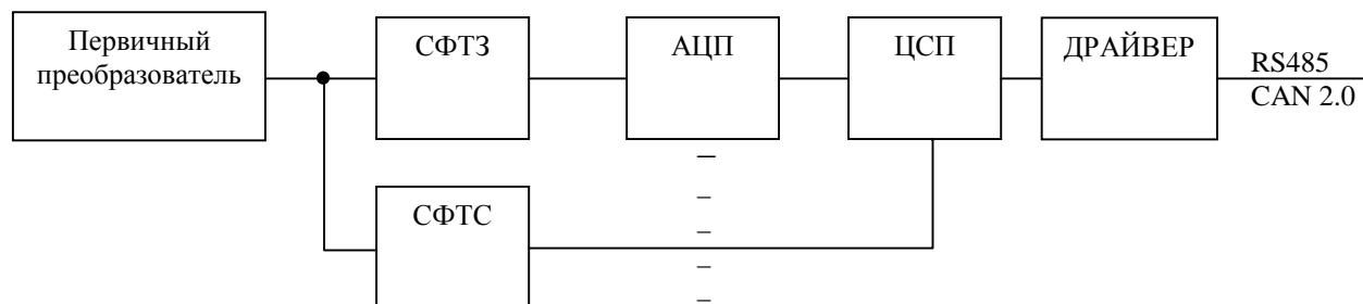
Рисунок 5 – Функциональная схема измерительного модуля
