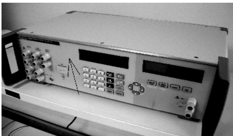
Рисунок 1 - Внешний вид калибратора в разных ракурсах. Стрелкой показано место нанесения знака утверждения типа.
