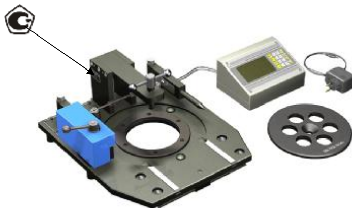
Рисунок 2 - Внешний вид приборов для контроля радиального и осевого зазоров подшипников модель БВ-7602-34 и место нанесения знака утверждения типа.
