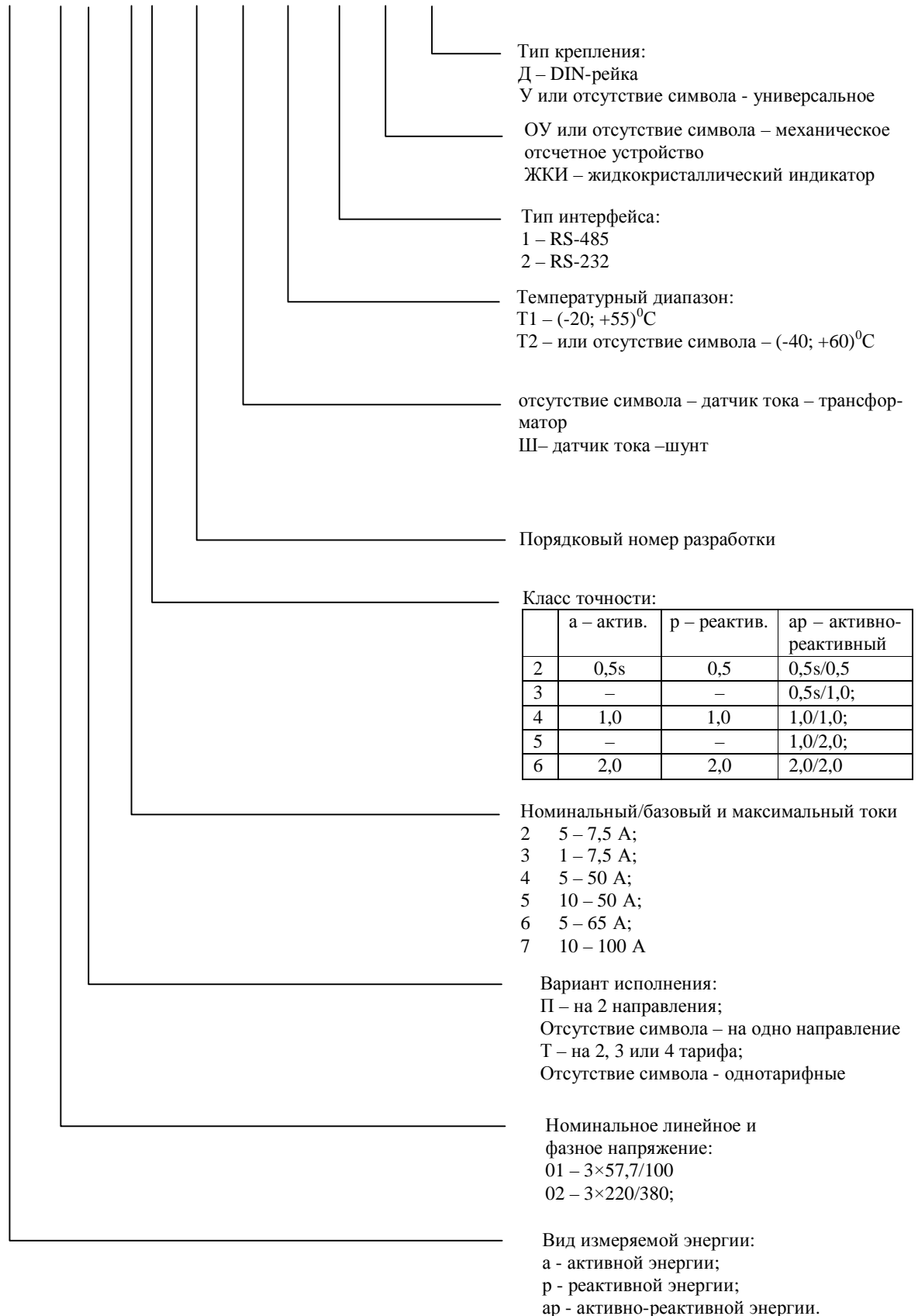
Рисунок 1 Структура условного обозначения счетчиков
