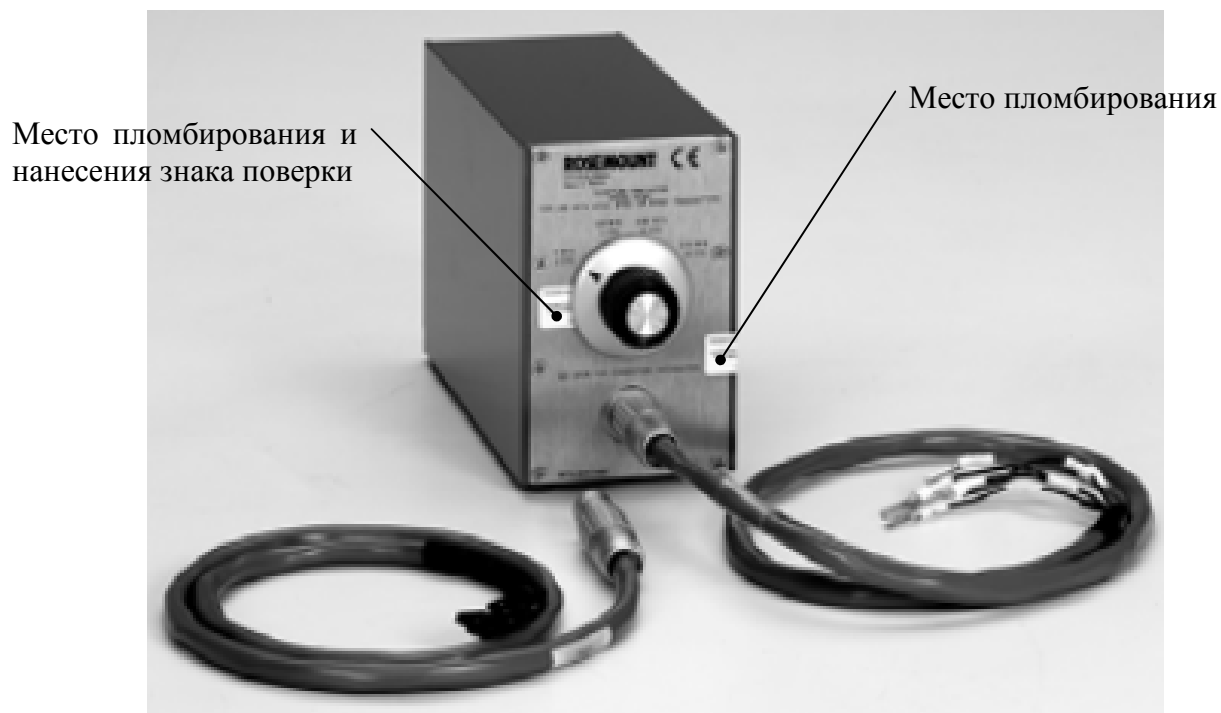
Рисунок 1 – Внешний вид имитатора 8714
