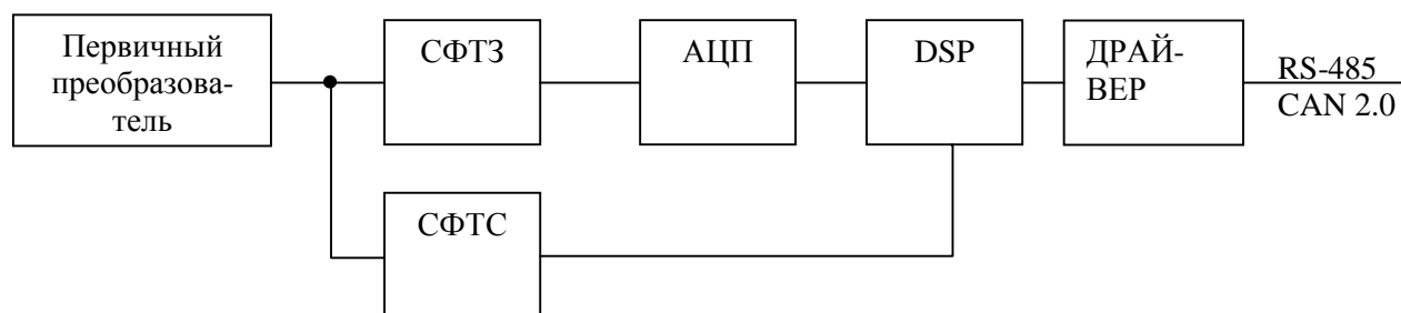
Рисунок 1 – Функциональная схема цифрового модуля
