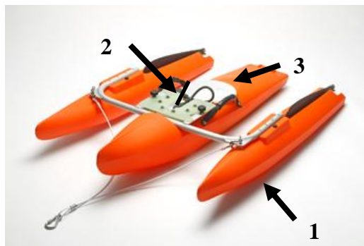
Рис.1 Внешний вид комплексов River Ray: 1 - тримаран; 2 - антенны блока связи; 3 - профилограф.
