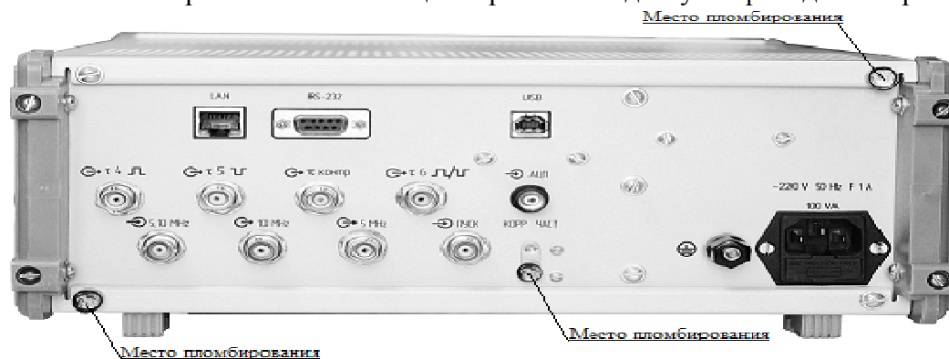
Рис. 2 Схема пломбирования прибора.
