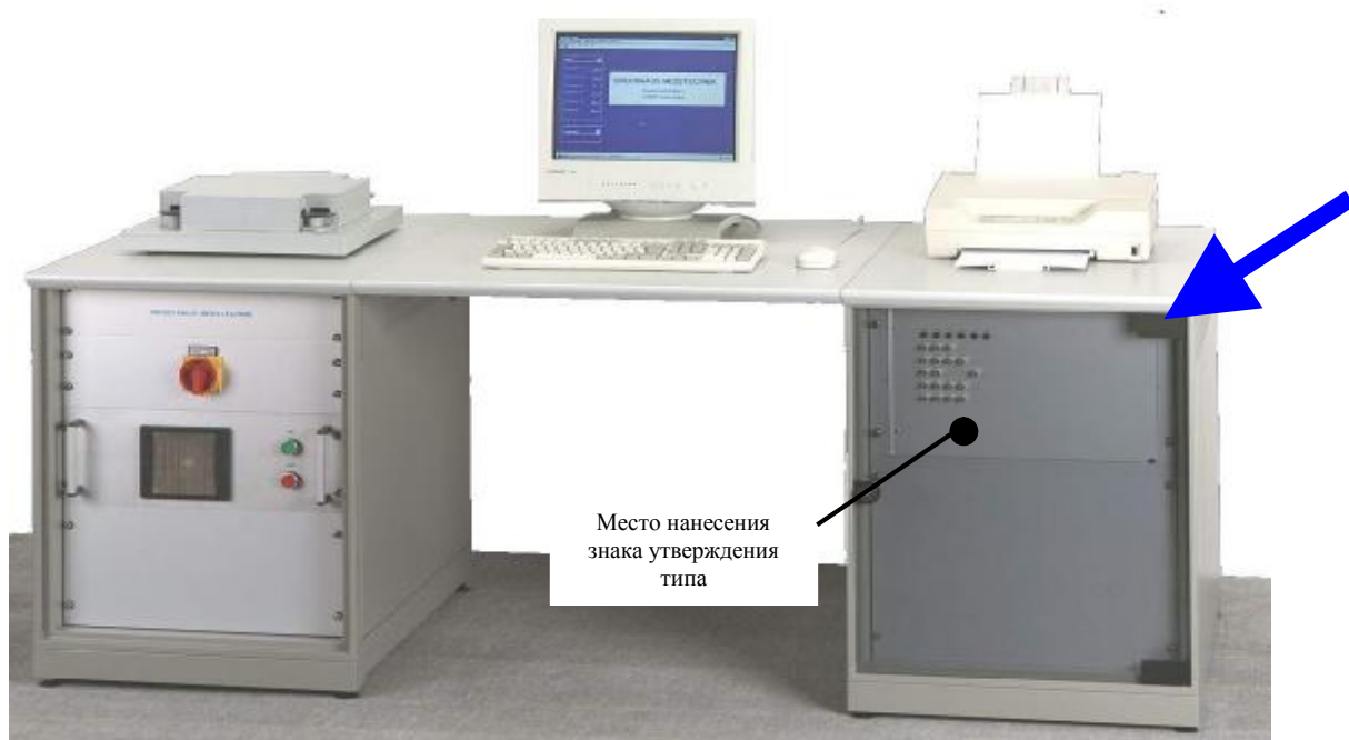
Рисунок 3 – Общий вид установки магнитоизмерительной MPG 100 D
