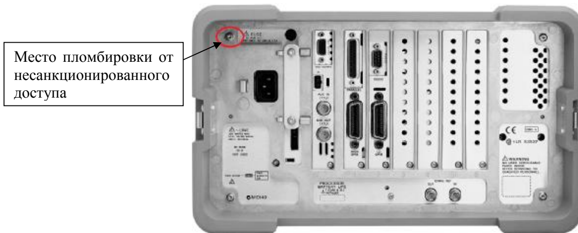
Рисунок 2. - Внешний вид измерителей N897XA. Задняя панель
