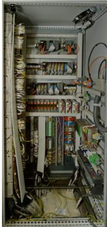
Рисунок 1 – Шкаф ИС САУ ДГУ
