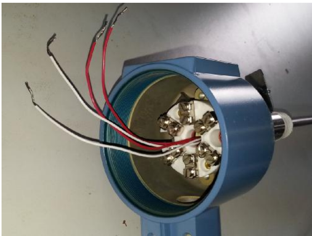
Рис. 1 – Термопреобразователь сопротивления платиновый Rosemount исполнения 0078D21A30B075T26
