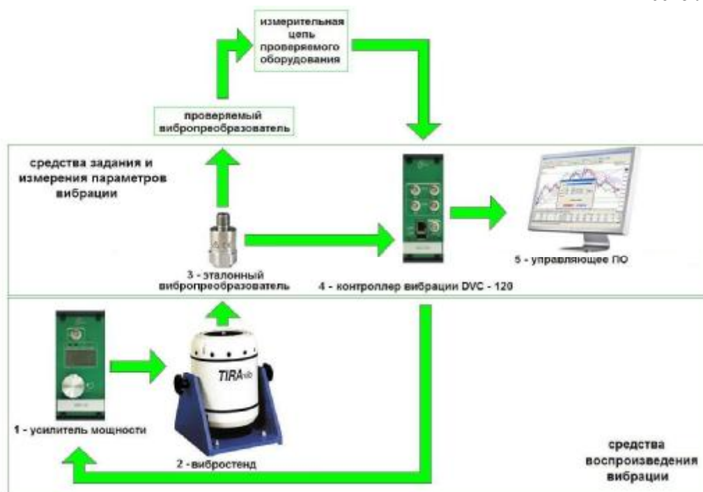
Рисунок 1 – Структурная схема виброустановки поверочной DVC-500
