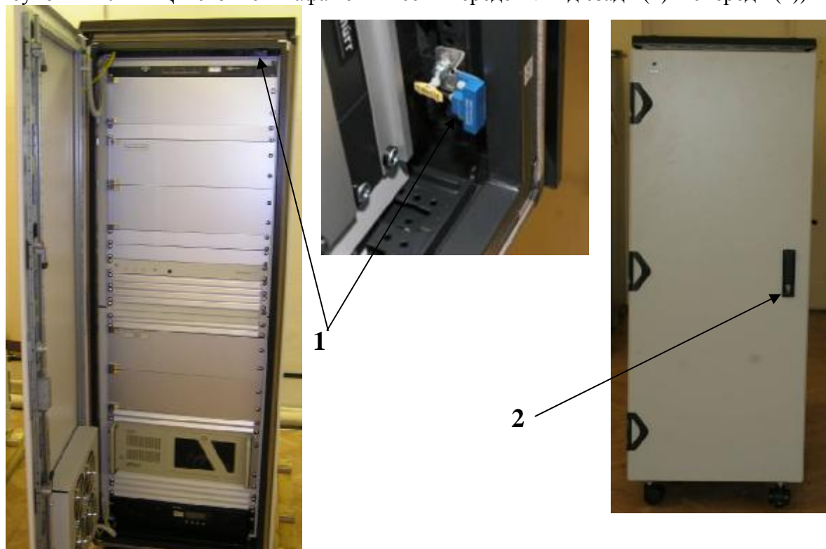
Рисунок 2 – УИ-ГЦ в стойке шкафа технических средств: вид сзади (1) и спереди (2))
