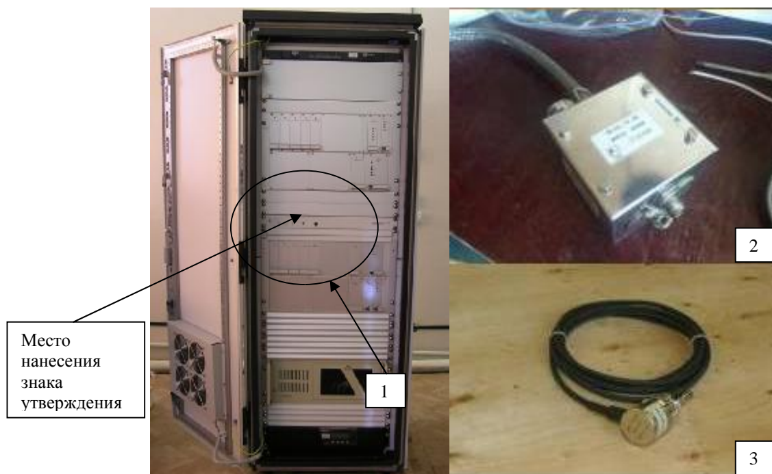
1 - Устройство информационно-измерительное УИ-14ВЦ (в стойке шкафа технических средств); 2 - Коммутационная коробочка КК-В; 3 - Зонд выносной СКТВ-ЗВ
