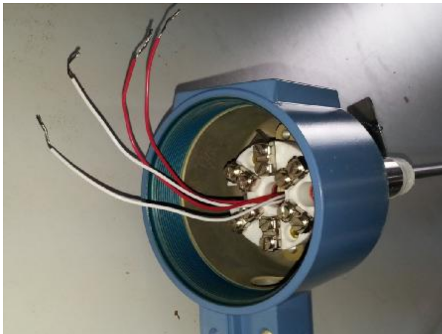
Рис. 1 – Термопреобразователь сопротивления платиновый Rosemount исполнения 0078D21A30B045T26
