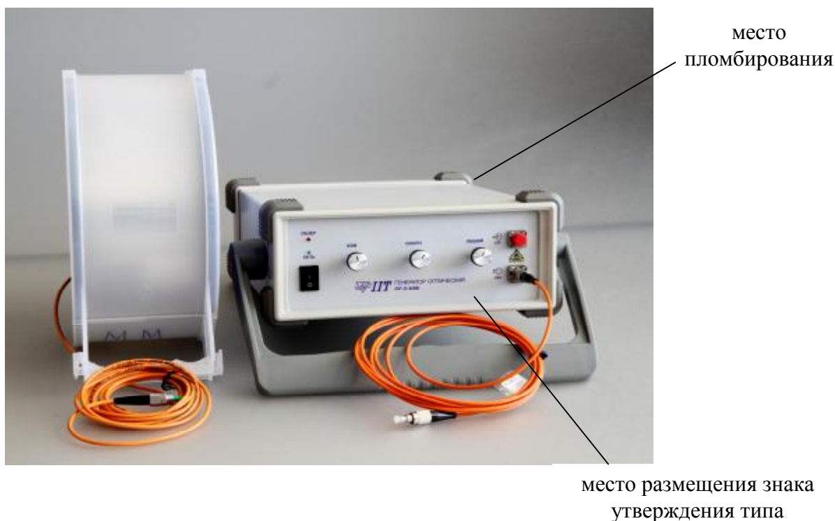
Рисунок 1 – Внешний вид рабочего эталона единиц длины и ослабления в световоде с указанием мест пломбирования и размещения знака утверждения типа
