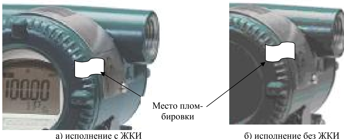
Рис. 4. Места пломбировки преобразователей (датчиков) давления измерительных ЕЖ*
