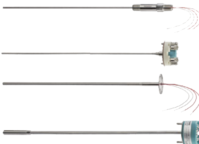
Рис.5 SITRANS TSinsert
