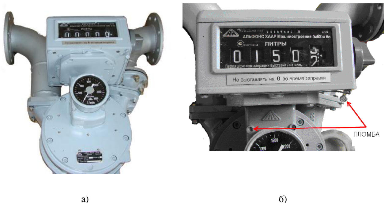
Рисунок 1 - Счетчики жидкости лопастные МКА Master
