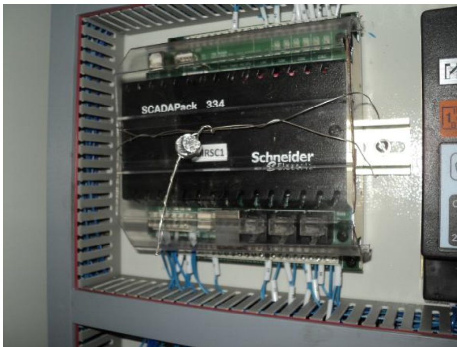
Рисунок 2 - Пломбировка корпуса контроллера SCADAPack (вид спереди)
