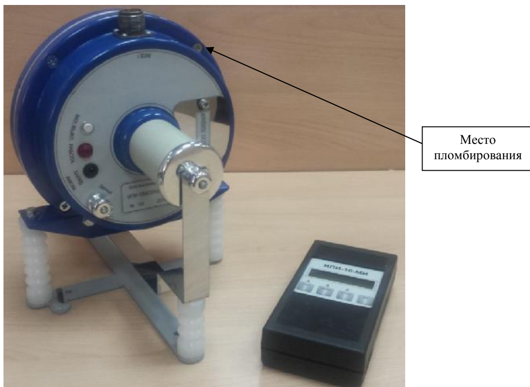
Рисунок 1 – Внешний вид и место пломбирования ИПИ-10-МОЛНИЯ-БВ
