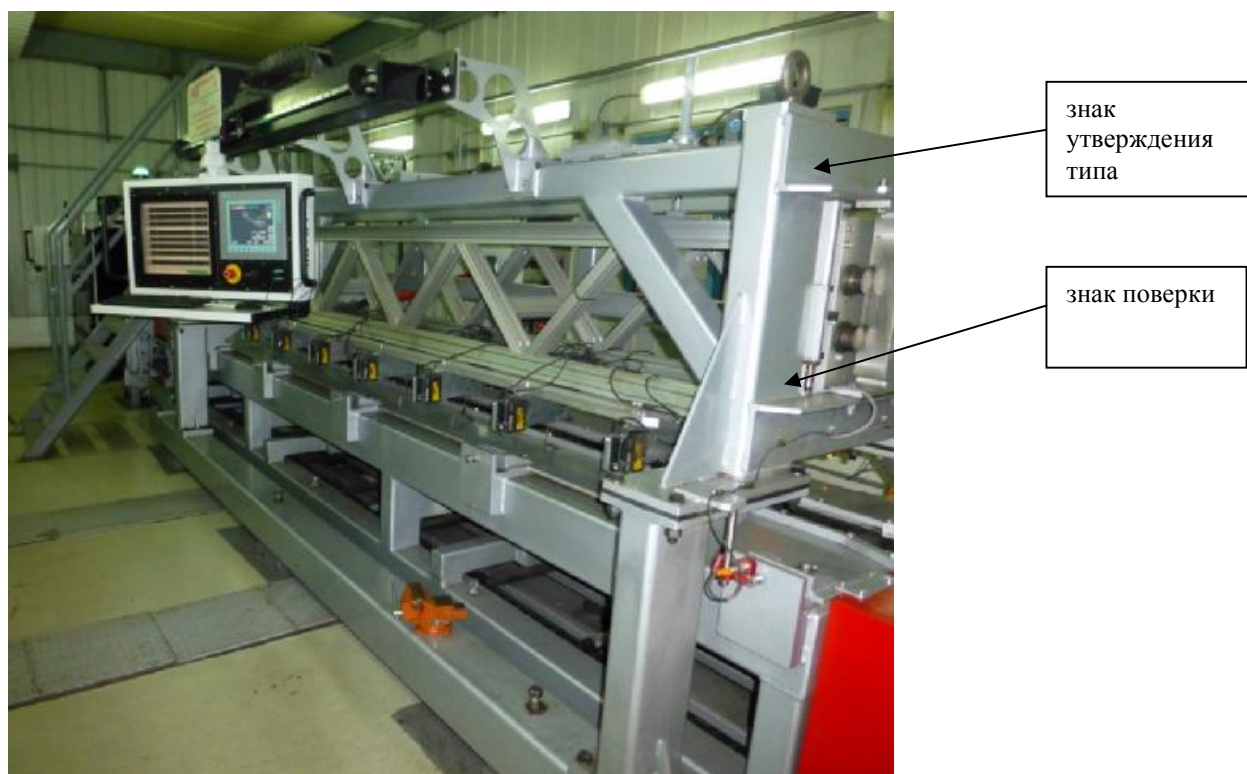
Рисунок 1 - Общий вид системы измерений отклонения от прямолинейности металлопрокатной продукции RSAS-800 и мест нанесения знаков утверждения типа и поверки
