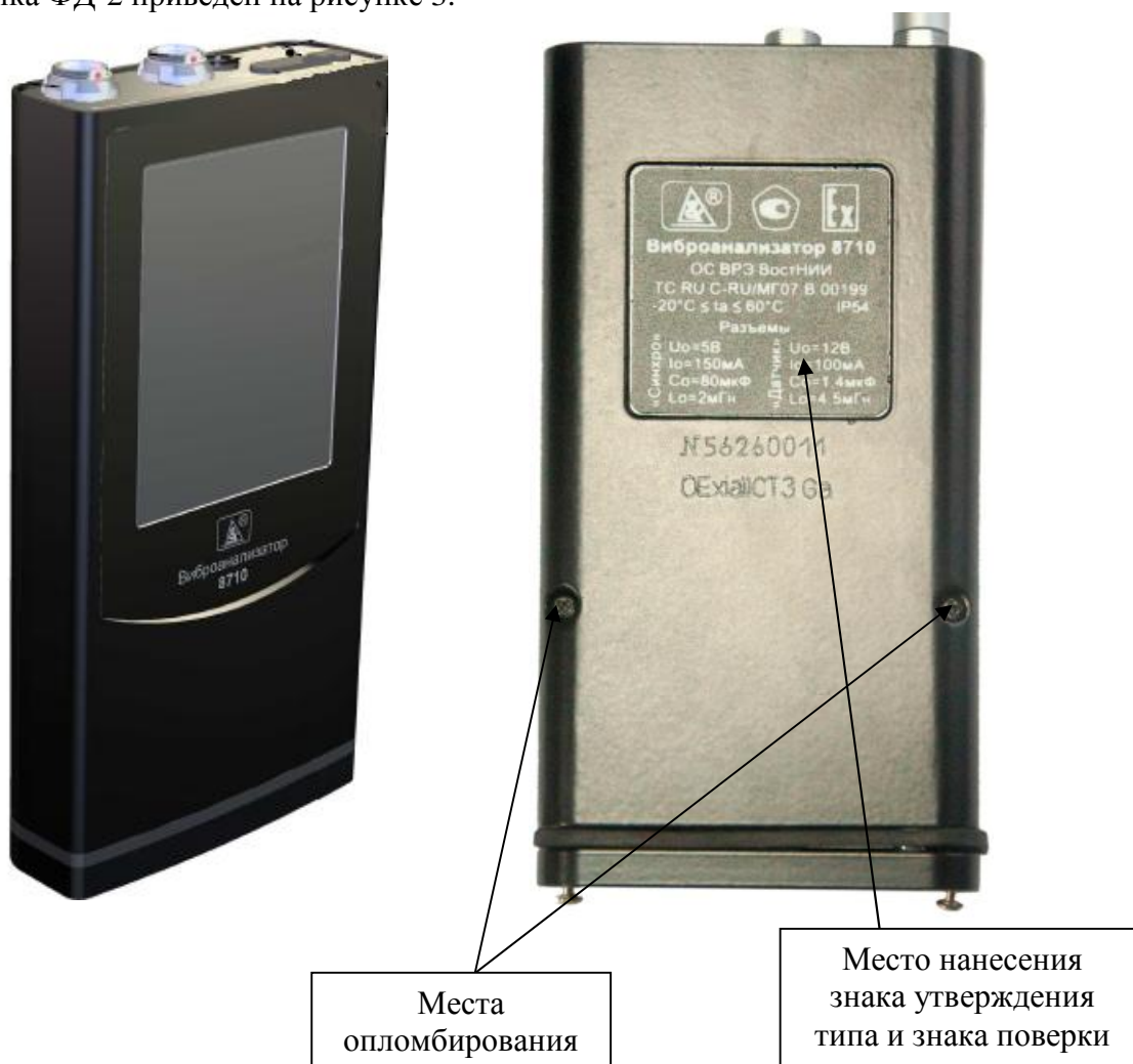
Рисунок 1 - Внешний вид вибронализатора 8710
