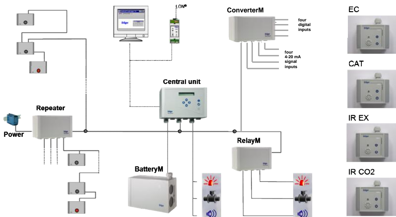
Рисунок 3 – Структурная схема Системы
