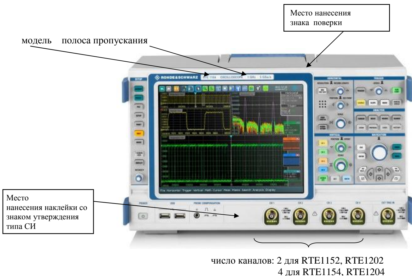
Рисунок 1 - Внешний вид осциллографов цифровых запоминающих RTE1152, RTE1154, RTE1202, RTE1204
