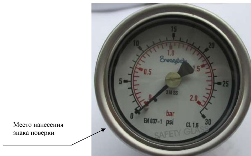
Рисунок 1 - Манометр показывающий PGI-63B-PG30
