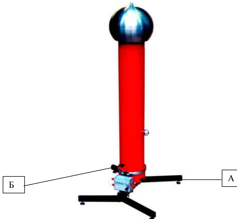
Рисунок 1 – Внешний вид делителя напряжения ДН-220пт Место пломбировки от несанкционированного доступа (А) и нанесения знака поверки (Б)
