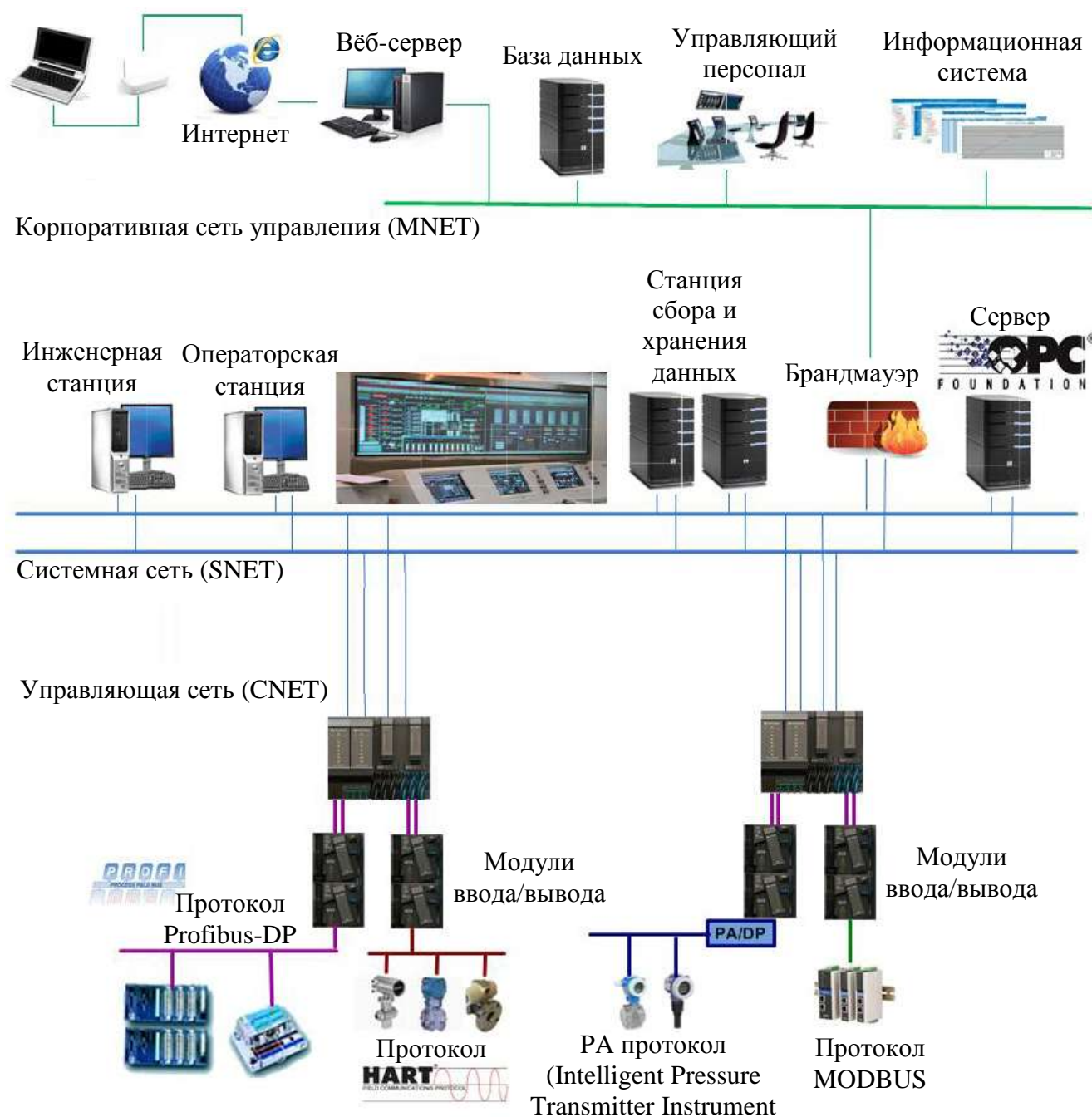
Рисунок 1 - Архитектура системы HOLLiAS MACS
