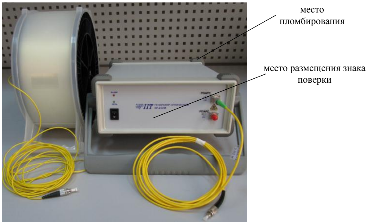
Рисунок 1 - Внешний вид рабочего эталона единиц длины и ослабления в световоде с указанием мест пломбирования и размещения знака поверки
