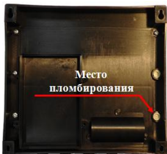
Рисунок 7 – Пломбирование тепловычислителя СПТ943
