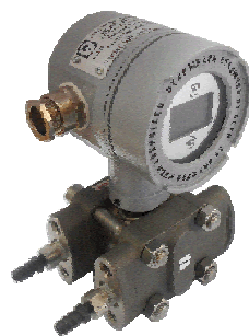
Рисунок 10 Датчик давления «ГиперФлоу», модель ДП-022
