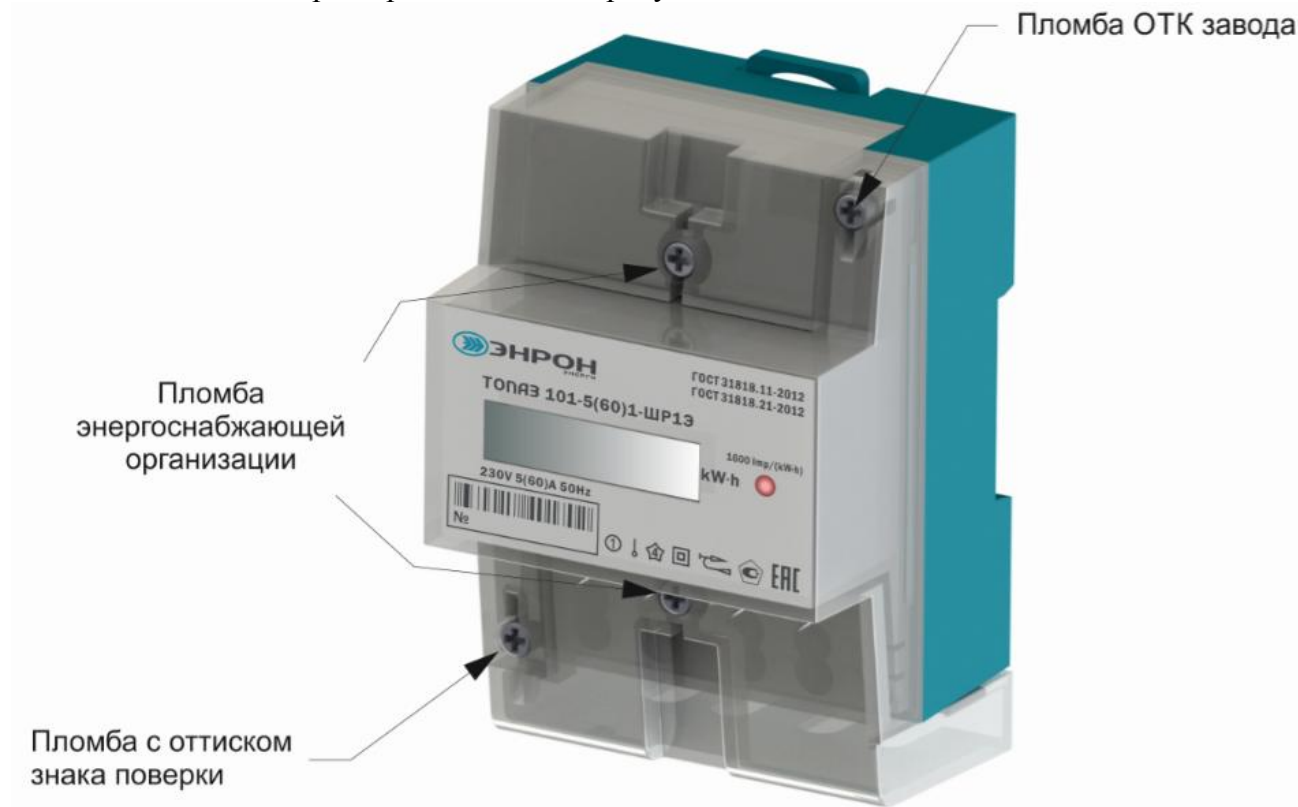
Рисунок 2 – Общий вид модификации счетчика ТОПАЗ 101
