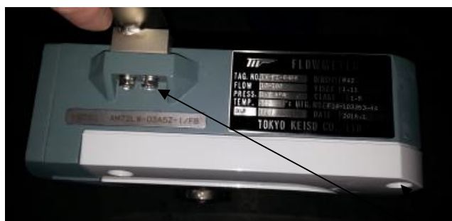
Рисунок 1 - Общий вид ротаметров AM72LW
