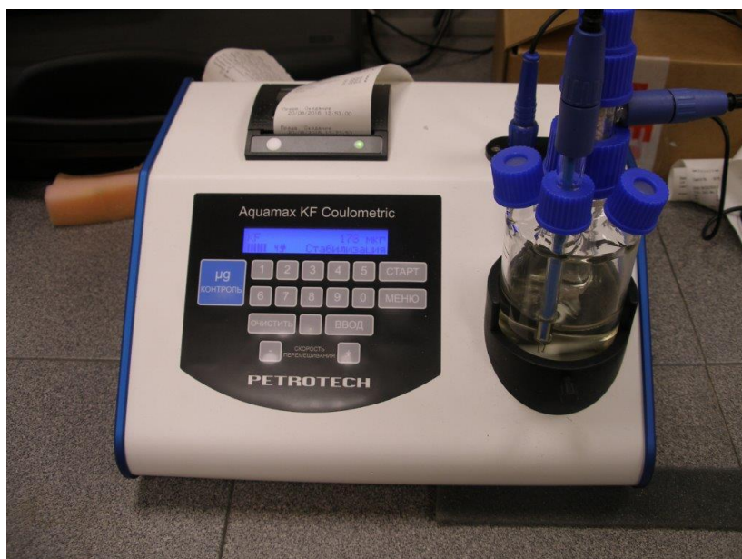
Рисунок 1 - Анализатор влажности кулонометрический Aquamax KF
