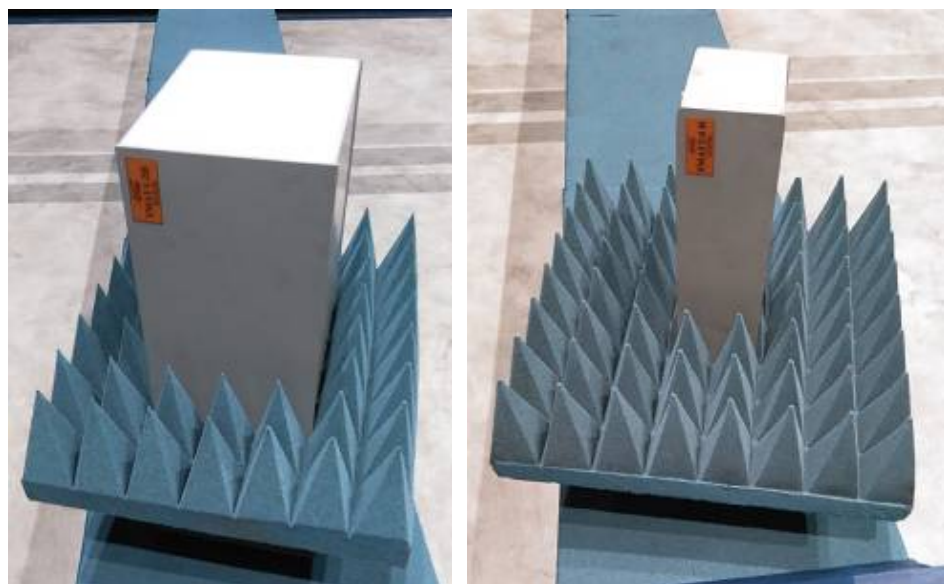
Рисунок 7 - Внешний вид антенн-зондов диапазона частот от 1 до 4 ГГц
