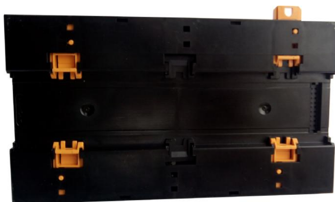
Рисунок 3 - Крепления преобразователя на DIN-рейке
