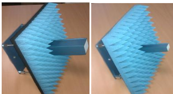
Рисунок 6 - Внешний вид антенн-зондов диапазона частот от 4 до 18 ГГц
