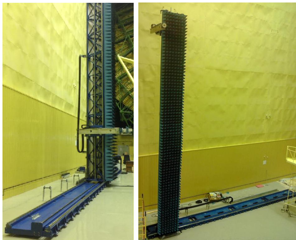
Рисунок 1 - Внешний вид сканера
