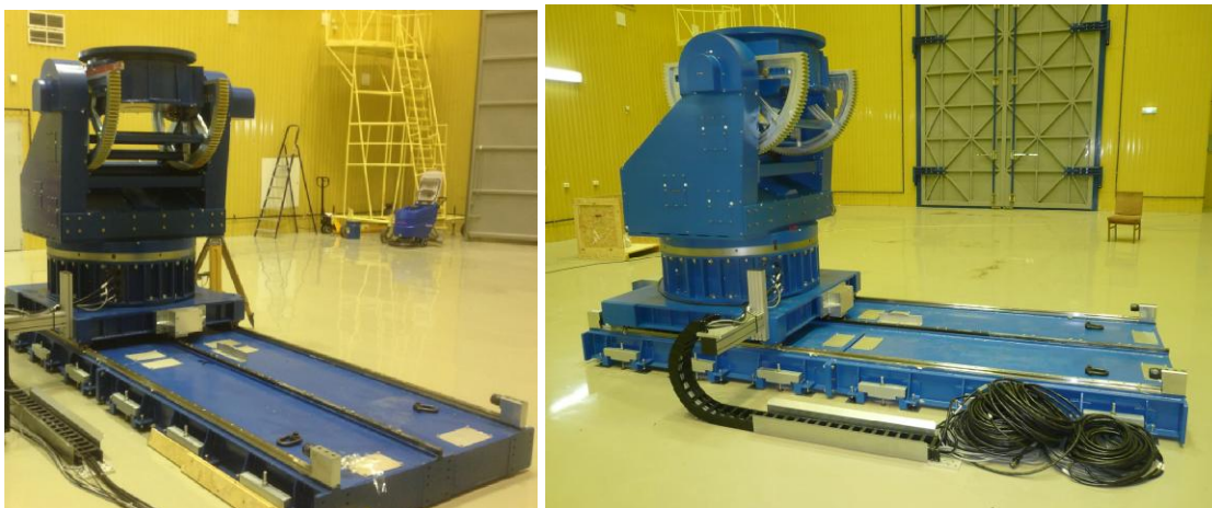
Рисунок 3 - Внешний вид ОПУ
