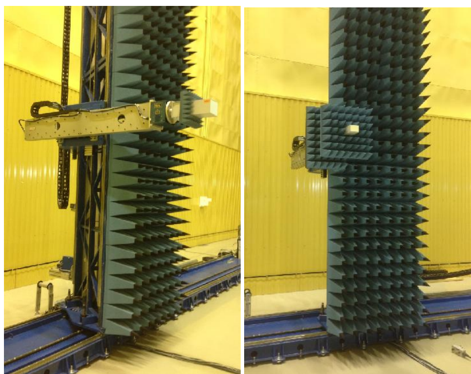
Рисунок 2 - Внешний вид сканера с установленной антенной-зондом
