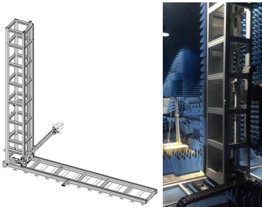
Рисунок 1 - Конструкция и общий вид сканера
